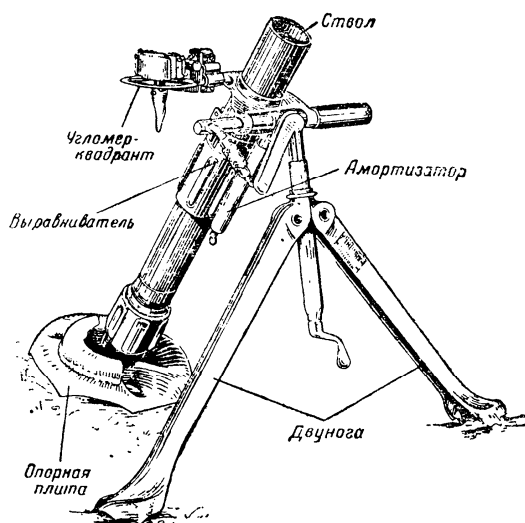
Рис. 16. 50-мм ротный миномет обр. 1940 г.
